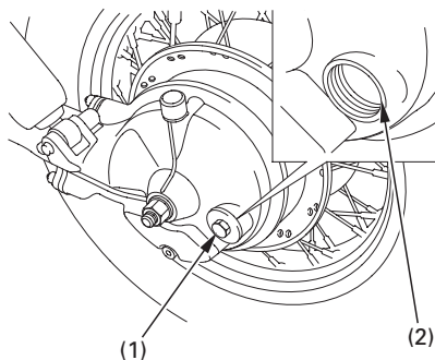
(1) Öljyn täyttötulppa (2) Öljyn täyttöaukko
